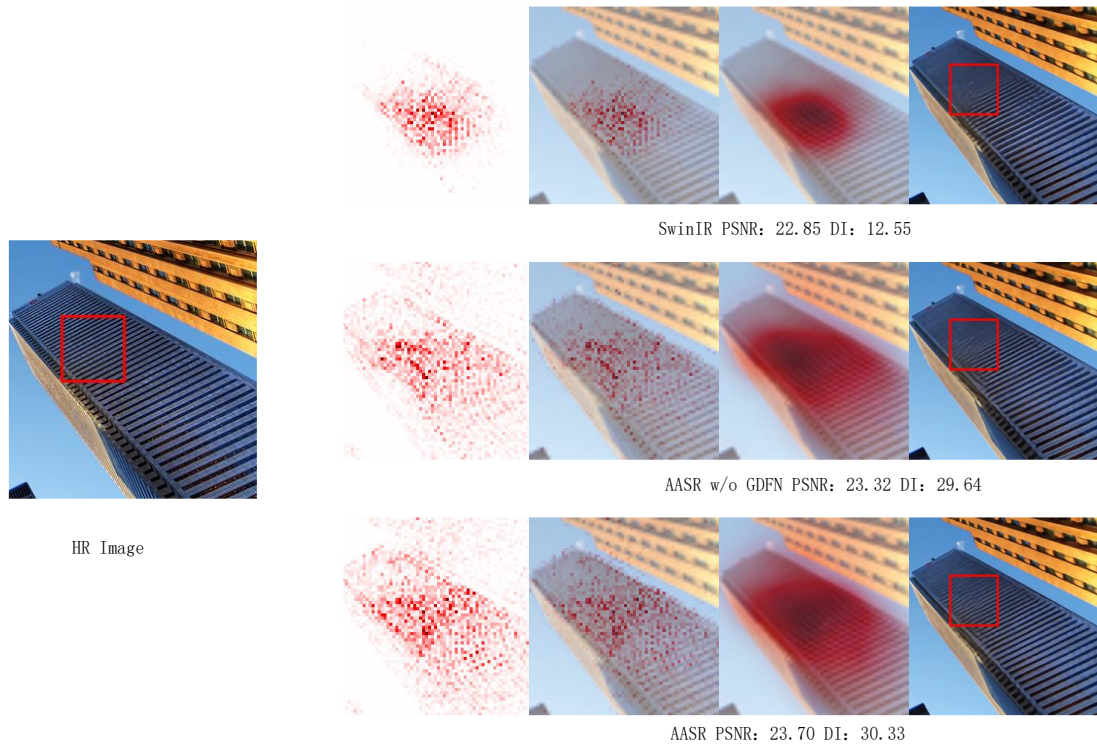
图 3-2 在 Urban100 img_012 上的 LAM 分析结果
